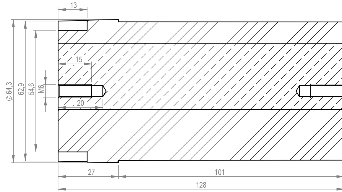
KESIT B-B
