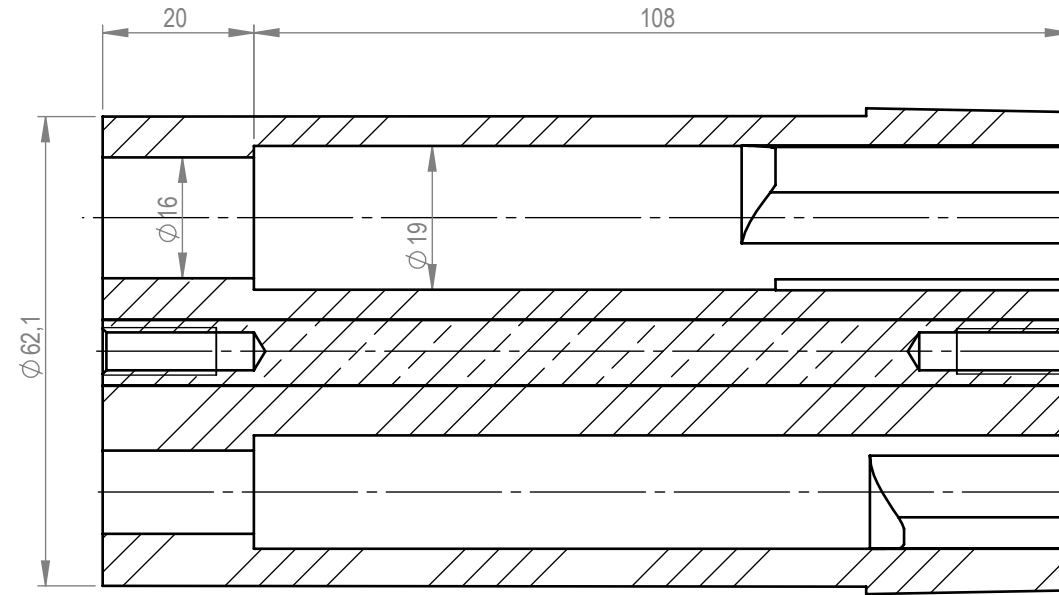
KESIT A-A
